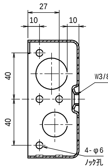
断面B-B
